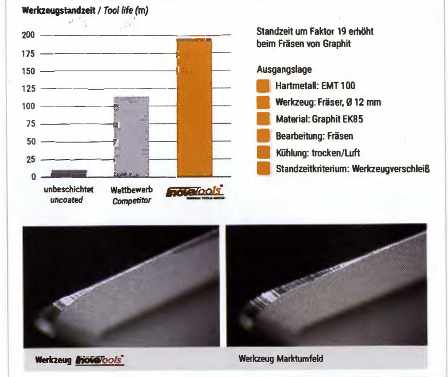
Verschleiß- und Standzeitvergleich.
